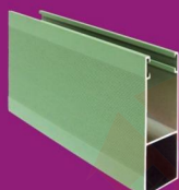
★xgd90#导槽-1.5 80#-0.8门片专用 颜色: 浅砂绿 Sand grain green
