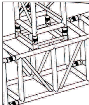
6.T字接头/T Corner
