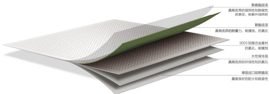
STRUCTURAL DRAWING 产品结构图
